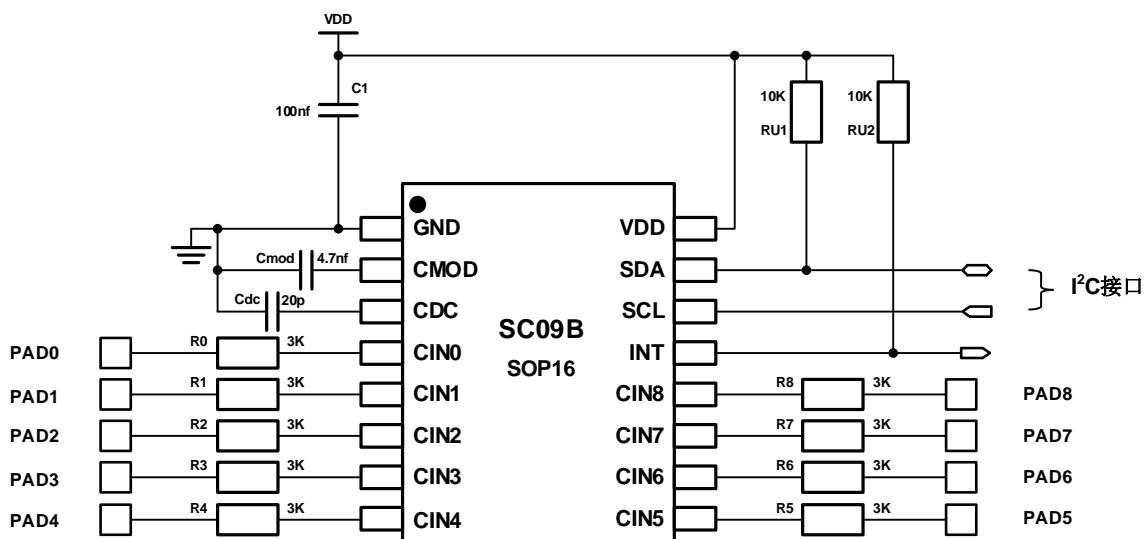
图3-1: 应用电路
