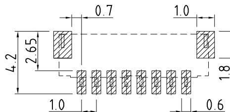
P.C.B LAYOUT
