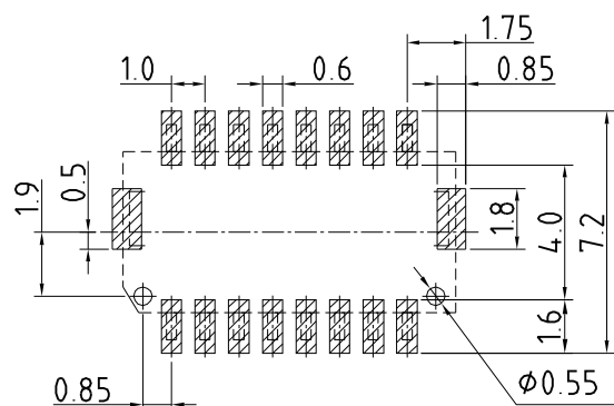
P.C.B LAYOUT
