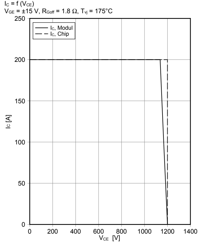
Sicherer Rückwärts-Arbeitsbereich IGBT, Wechselrichter (RBSOA) reverse bias safe operating area IGBT, Inverter (RBSOA) I_C = f(V_{CE}) V_{GE} = \pm 15\text{ V} , R_{Goff} = 1.8\ \Omega , T_{vj} = 175^\circ\text{C}
