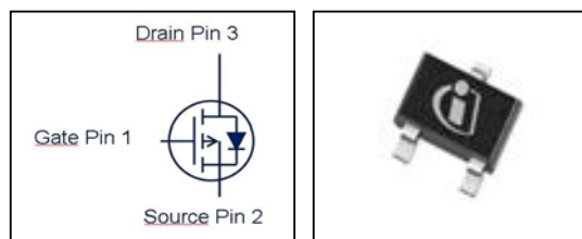
PG-SOT-323
