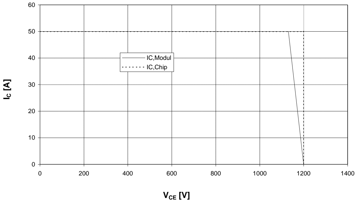
Sicherer Arbeitsbereich Wechselr. (RBSOA) I_C = f(V_{CE}) Reverse bias safe operating area Inverter (RBSOA) T_{vi} = 125^\circ\text{C} , V_{GE} = \pm 15\text{V} , R_G = 27\ \text{Ohm}
