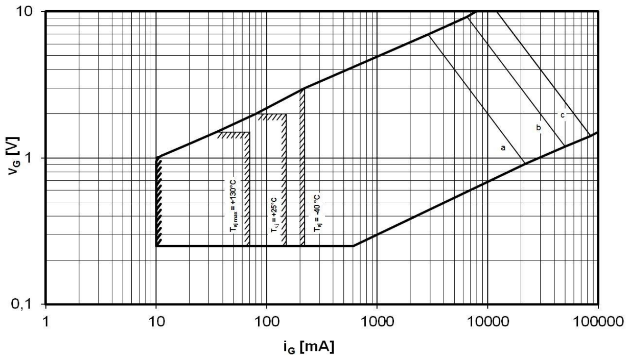
Steuercharakteristik v_G = f(i_G) mit Zündbereichen für V_D = 12 V Gate characteristic v_G = f(i_G) with triggering area for V_D = 12 V
