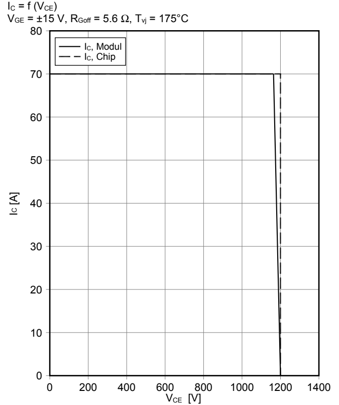
Sicherer Rückwärts-Arbeitsbereich IGBT, Wechselrichter (RBSOA) reverse bias safe operating area IGBT, Inverter (RBSOA) I_C = f(V_{CE}) V_{GE} = \pm 15\text{ V} , R_{Goff} = 5.6\ \Omega , T_{vj} = 175^\circ\text{C}
