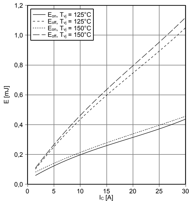
Schaltverluste IGBT,3-Level (typisch) switching losses IGBT,3-Level (typical)
