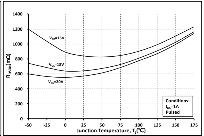
图. 6 各 V GS 下的 Ron 和温度关系曲线
