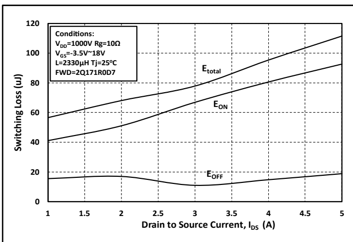
图. 21 开关能量和漏端电流 I DS 关系曲线
