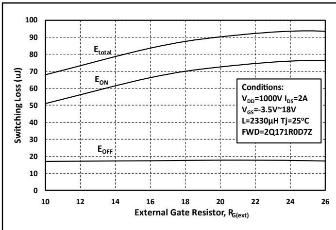
图. 19 开关能量和栅极电阻 R G(ext) 关系曲线
