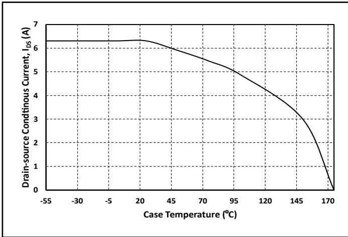
图. 23 漏端电流和温度关系曲线
