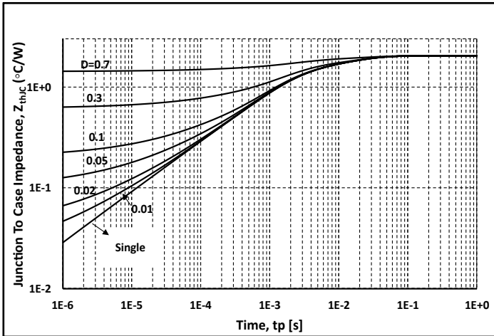
图. 25 热阻曲线
