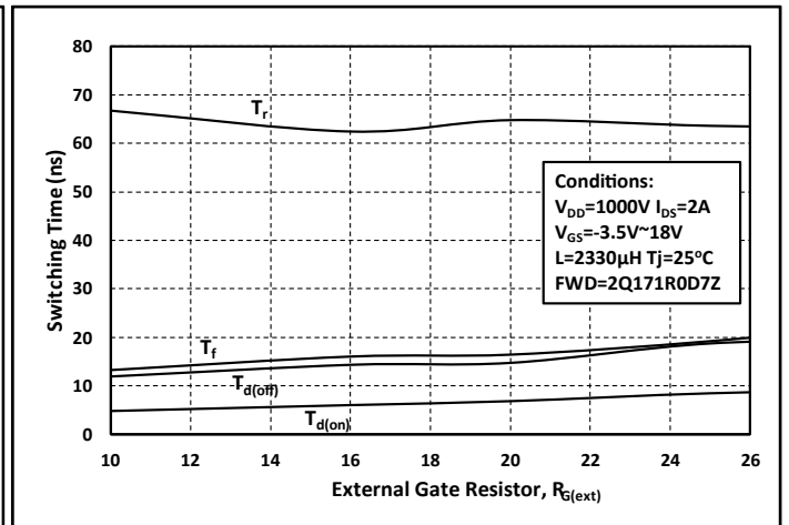
图. 20 开关时间和栅极电阻 R G(ext) 关系曲线
