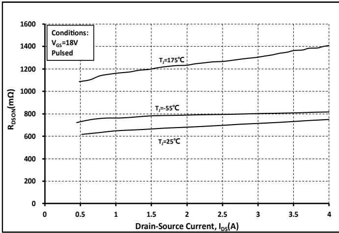
图. 5 各温度下的 Ron 和 I DS 关系曲线
