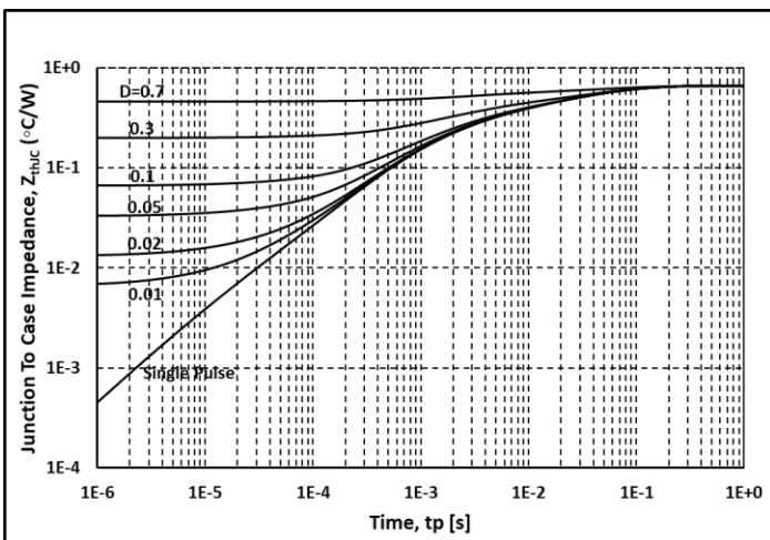
图. 23 热阻曲线
