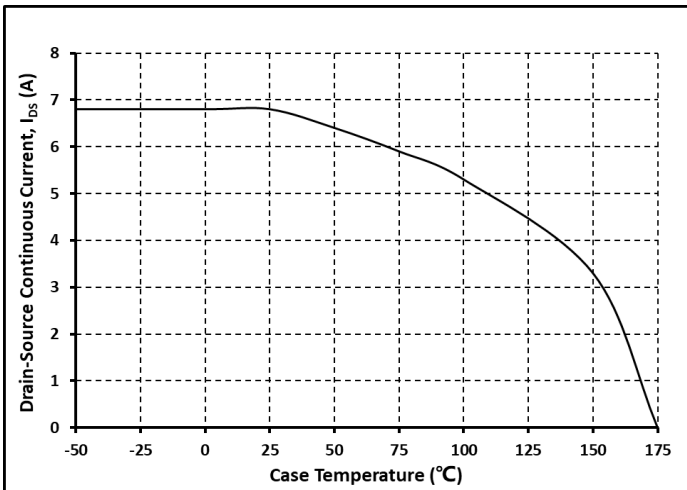
图. 21 漏端电流和壳温关系曲线
