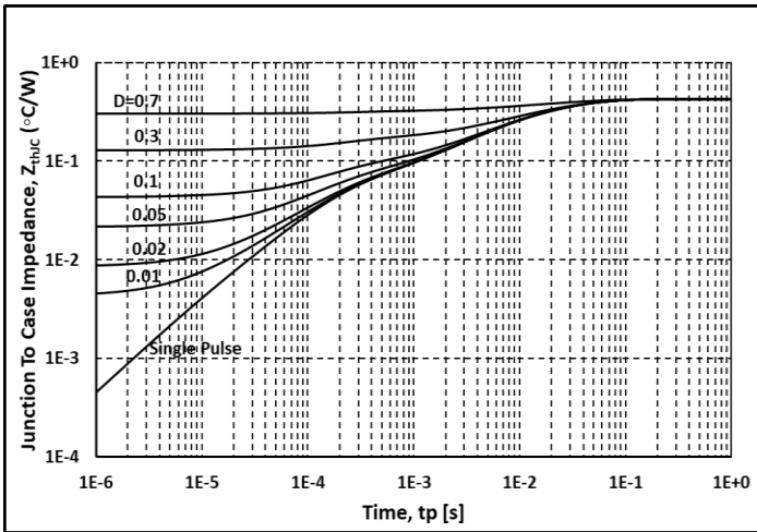
图. 25 热阻曲线
