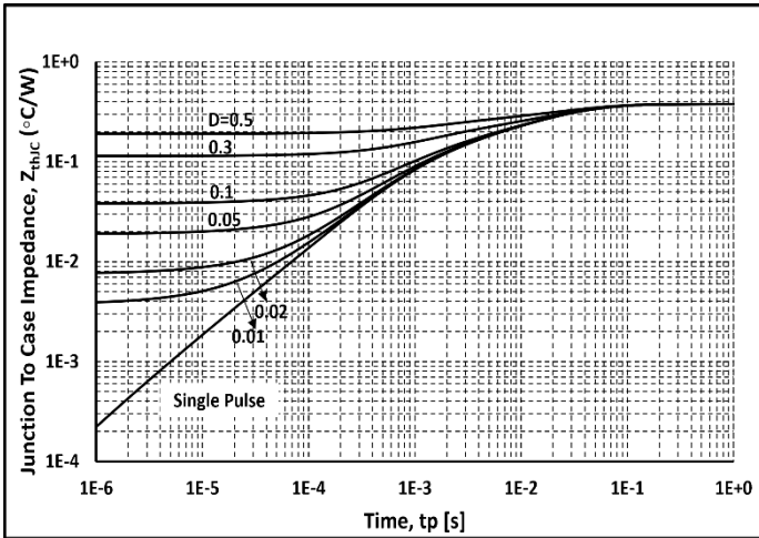
图. 25 热阻曲线
