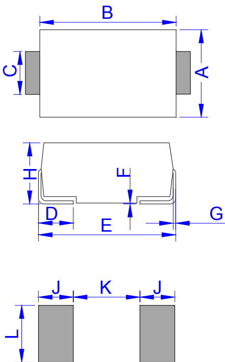
DO-214AB (SMC)
