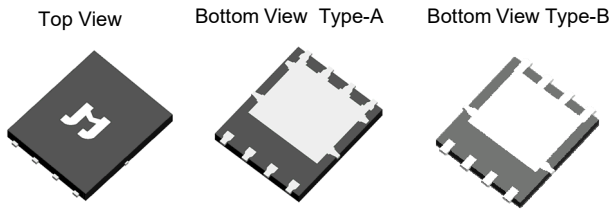
PDFN5x6-8L
