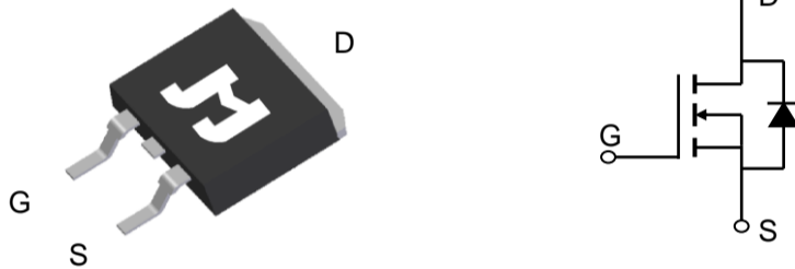
TO-263-3L Top View
