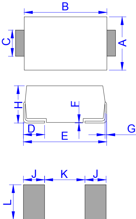
DO-214AB (SMC)
