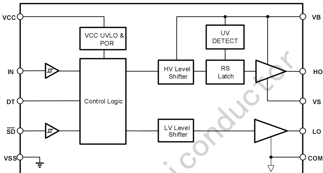
图7-1 TF21844M-TR功能框图
