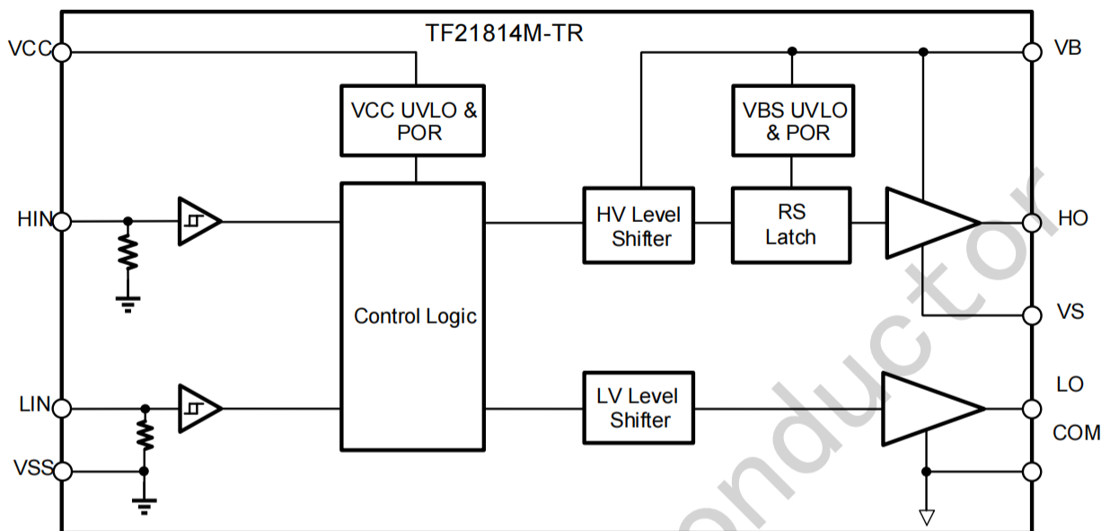
图7-1 TF21814M-TR功能框图
