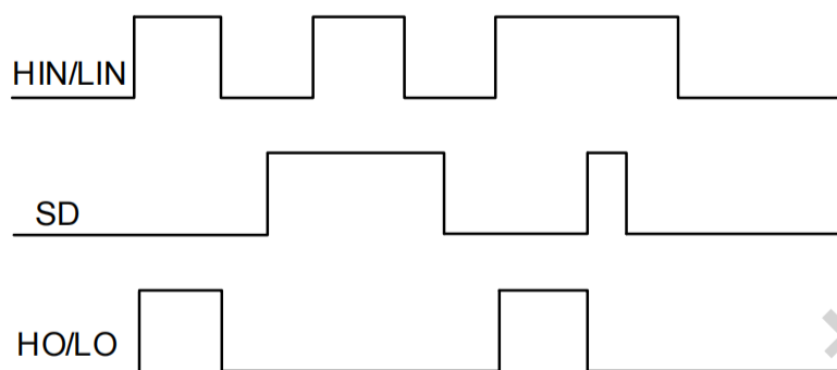
图 6-1 IR2113S输入输出时序波形
