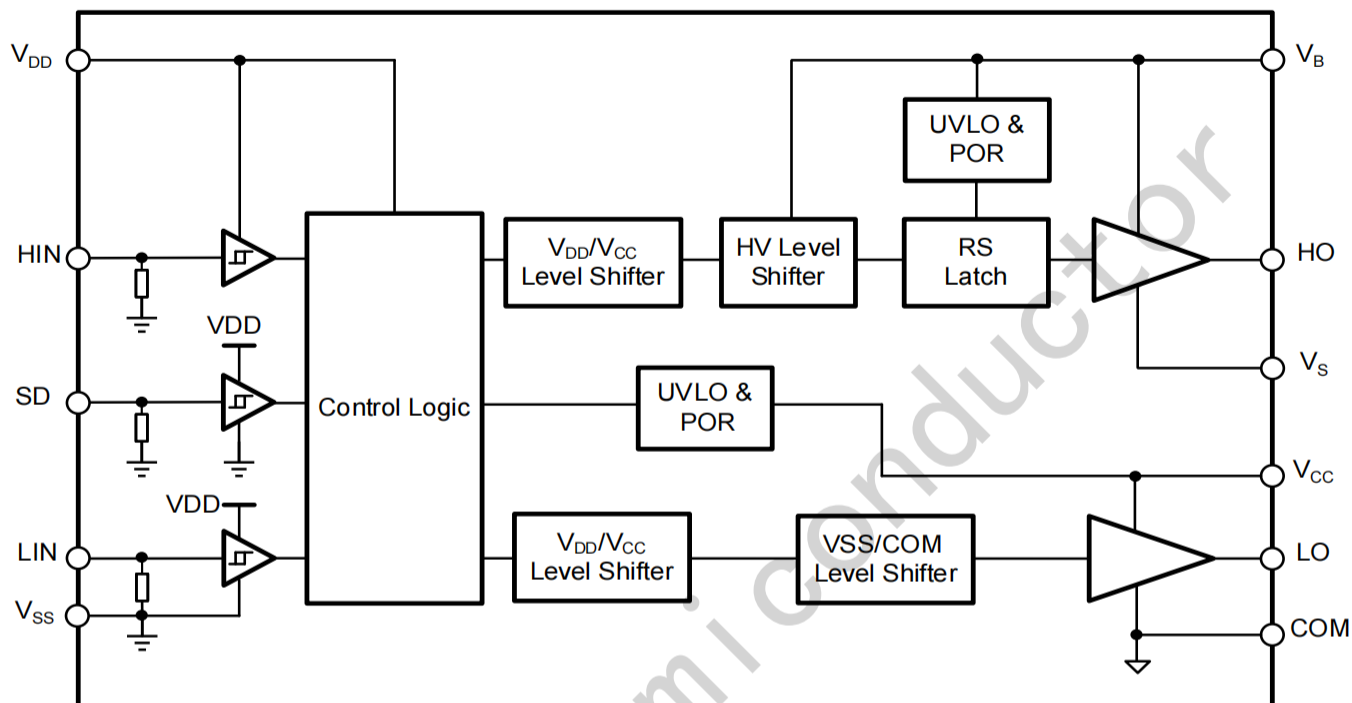
图 7-1 IR2113S功能框图
