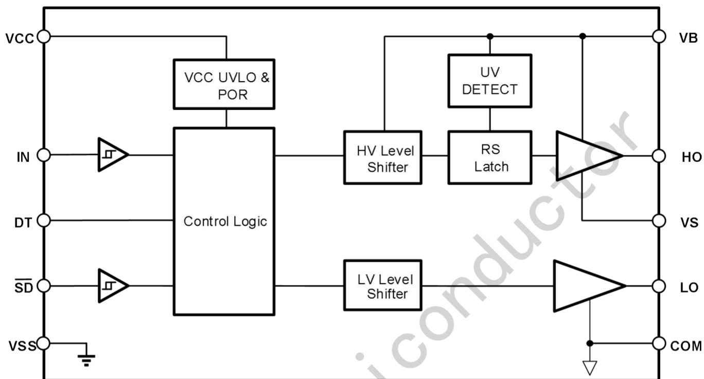
图7-1 LF21844NTR功能框图
