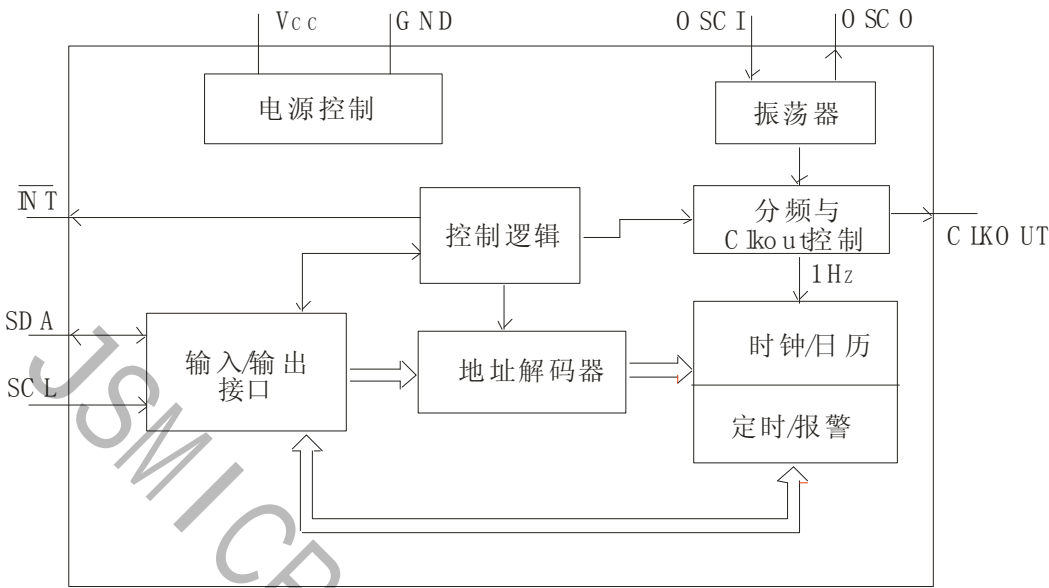
图 2. 方框图
