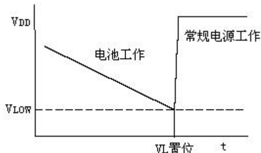
图8. 掉电检测
