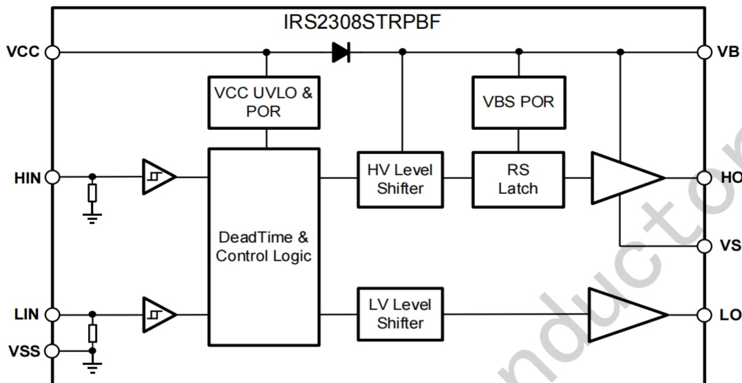
图7-1 IRS2308S的功能框图
