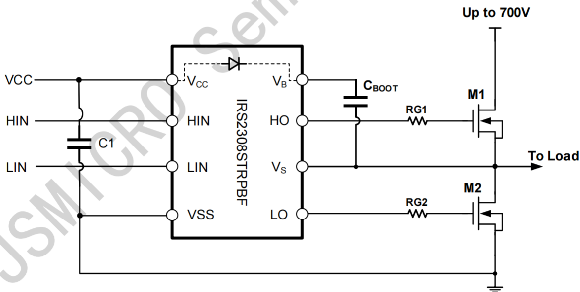
图7-2 IRS2308S典型应用电路图
