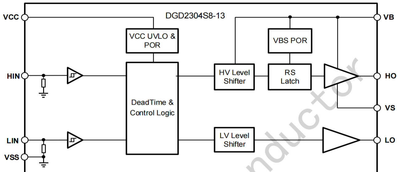
图7-1 DGD2304S8-13的功能框图
