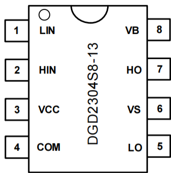
图4-1 SOP-8顶视图
