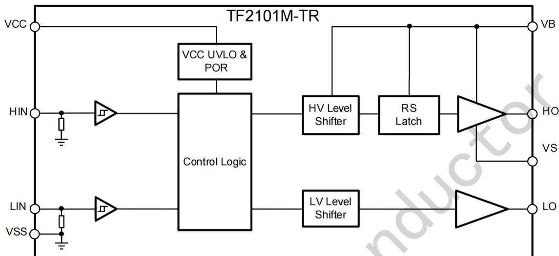
图 7 -1 TF2101M 的功能框图
