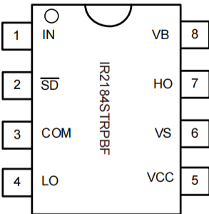
图4-1 8-脚SOIC顶视图
