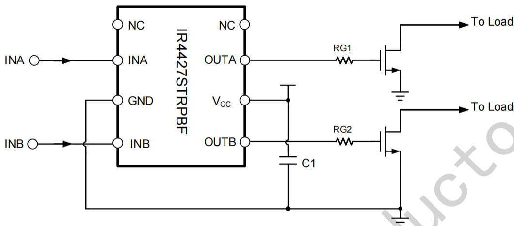
图 8-1 IR4427S典型应用电路图
