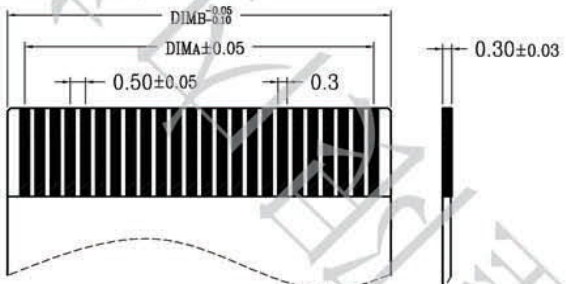
适用扁平线
