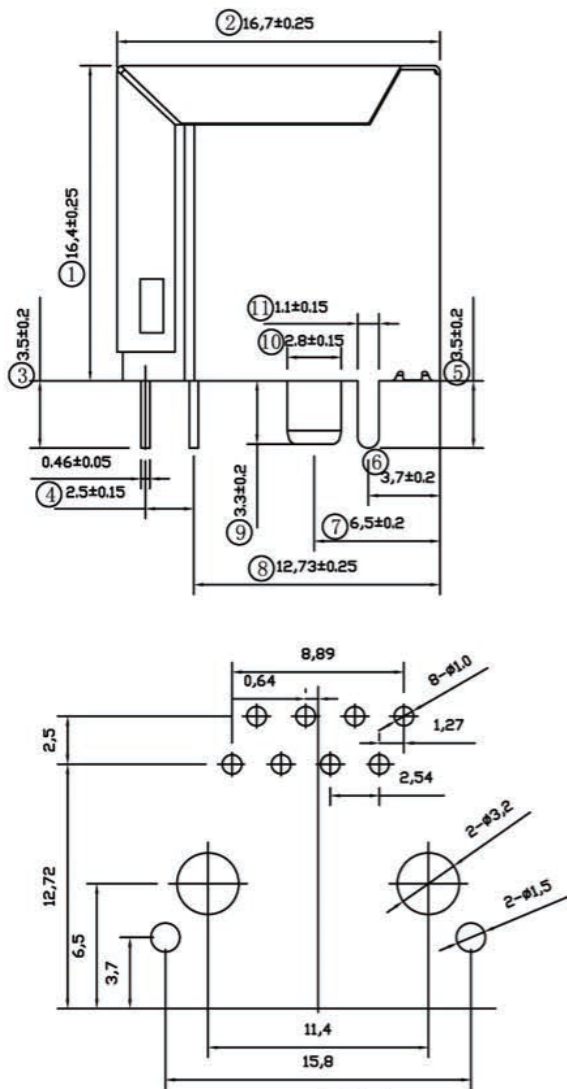
P. C. B参考图 (建议板后1.6mm)
