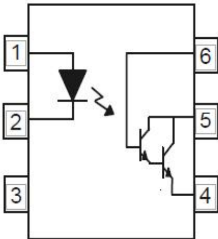
引脚配置 Pin Configuration
