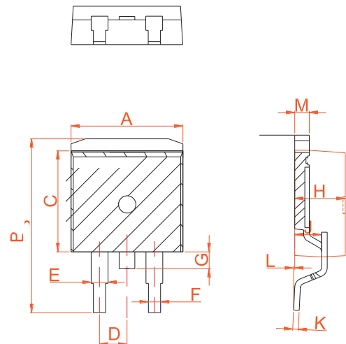
TO-263
