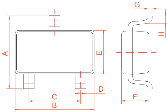
SOT-23-3L
