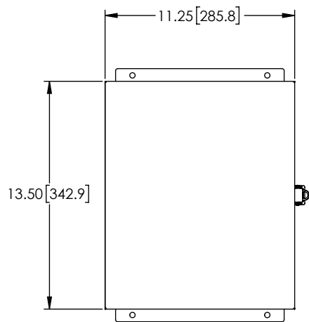
VIEW A-A
