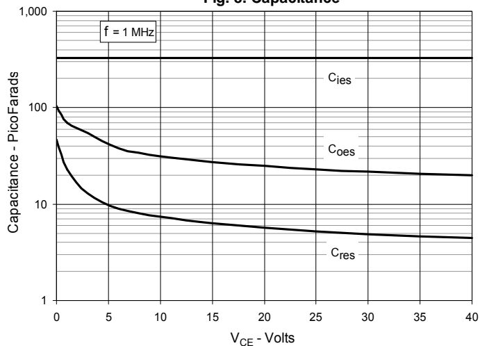
Fig. 8. Capacitance
