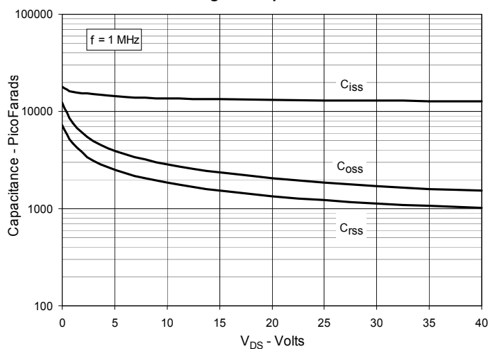
Fig. 11. Capacitance
