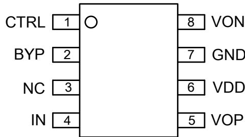
图 1. LPA2103 的管脚定义图
