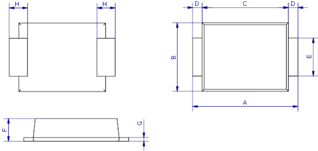
SMB-FL
