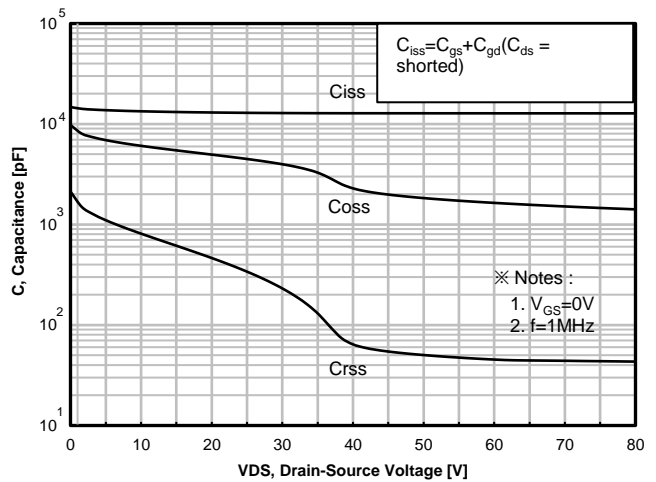
Fig. 8. Capacitance
