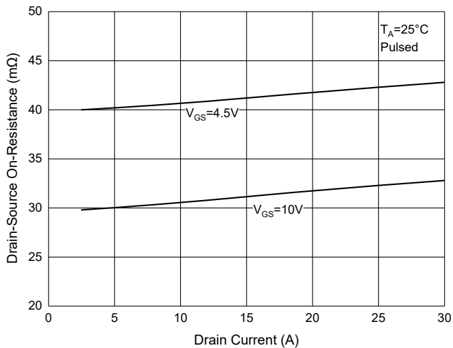
Fig. 5 - R_{DS(ON)} - I_D
