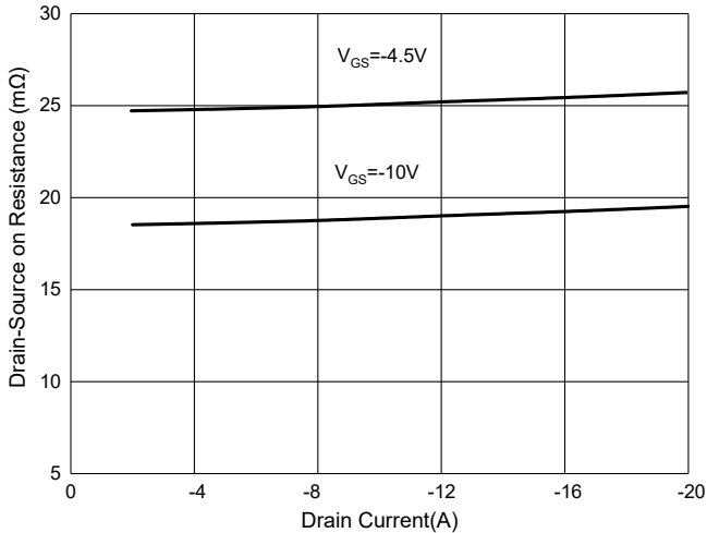
Fig. 10 - R_{DS(ON)} - I_D
