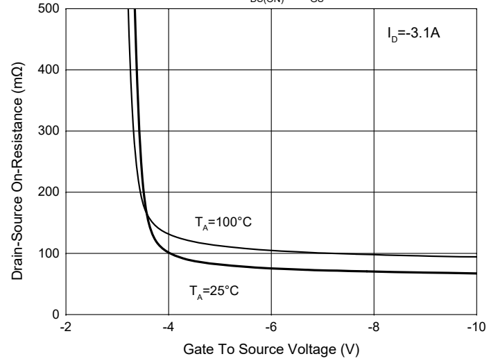
Fig. 4 - R_{DS(ON)} - V_{GS}
