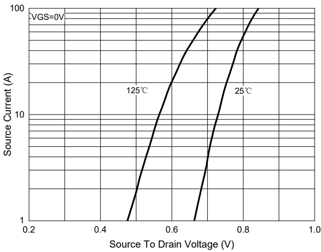
Fig.9 - I_s - V_{SD}
