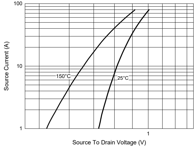
Fig. 8 - I_s - V_{SD}
