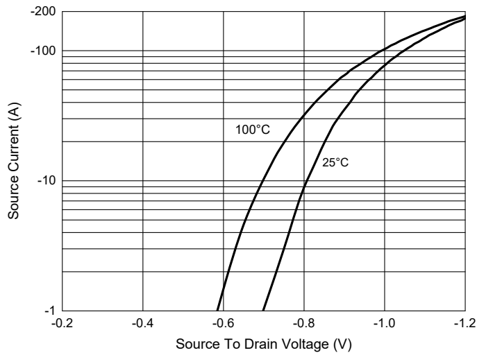
Fig. 7 - I_S - V_{SD}
