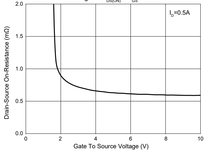
Fig. 2 - R_{DS(ON)} - V_{GS}
