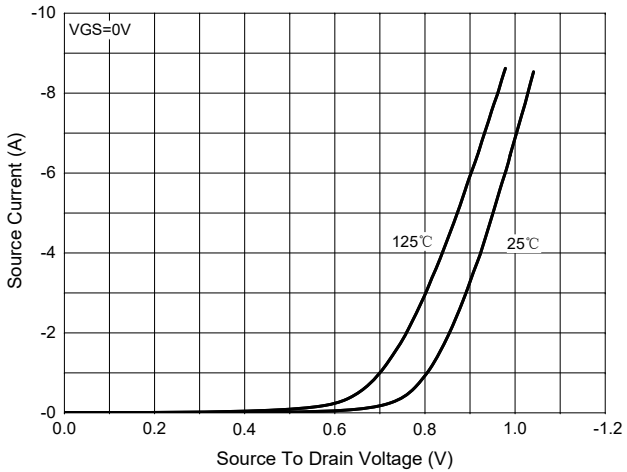
Fig. 5 - I_S - V_{SD}
