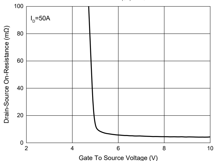
Fig. 6 - R_{DS(ON)} - V_{GS}
