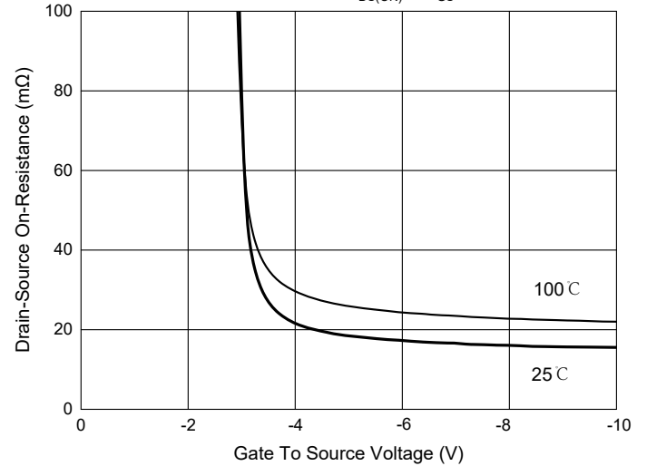
Fig. 6 - R_{DS(ON)} - V_{GS}
