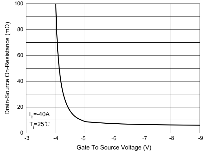
Fig. 8 - R_{DS(ON)} - V_{GS}
