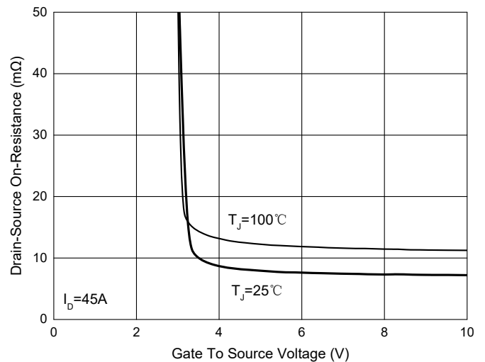
Fig. 6 - R_{DS(ON)} - V_{GS}
